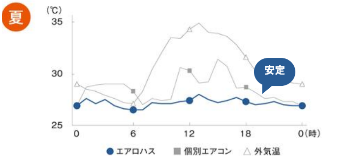
空調の違いによる1日の温度変化の比較 (LDKの場合)
